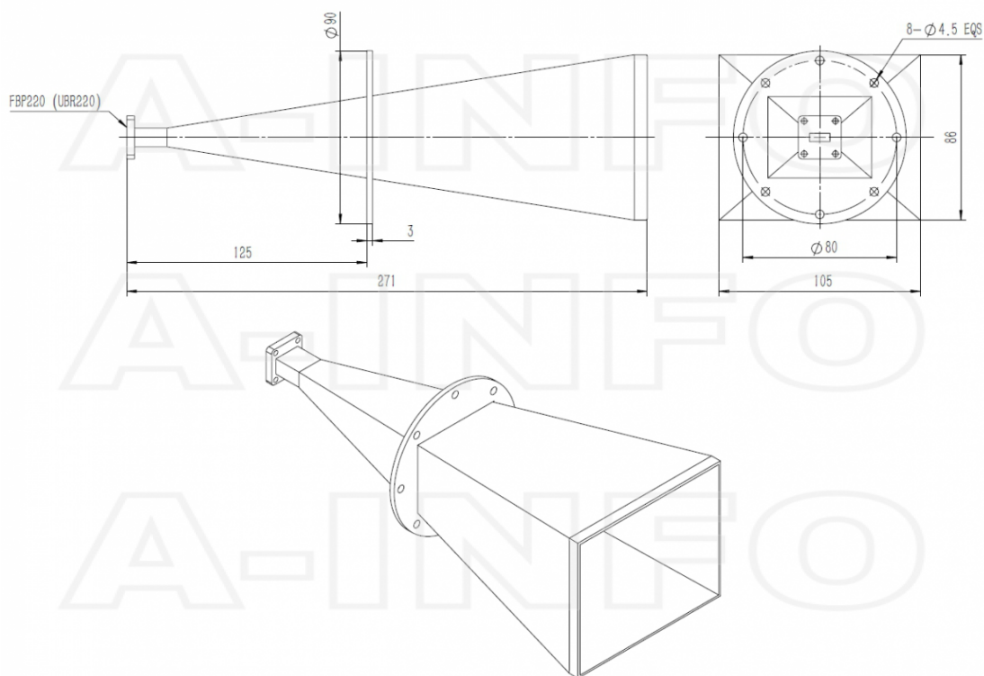
FBP220 Output (P/N: LB-42-25-A2)
